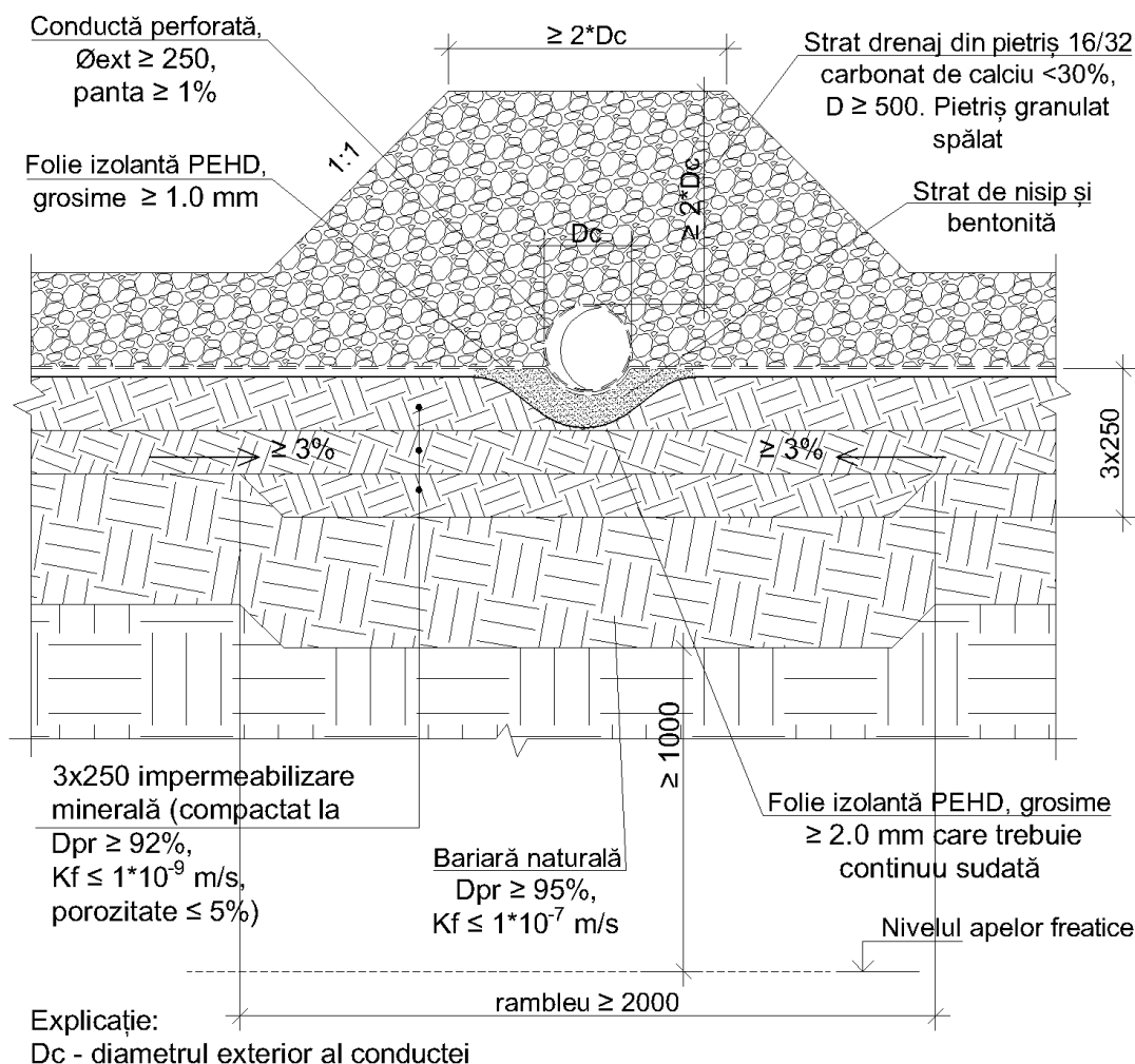
Figura 2 – Impermeabilizarea bazei pentru depozitele de deșeuri nepericuloase
