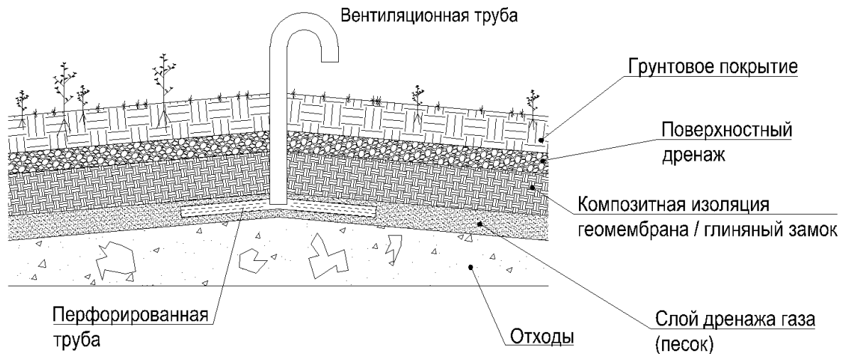
Рисунок 7 - Схема отведения газа через слой окончательного покрытия
