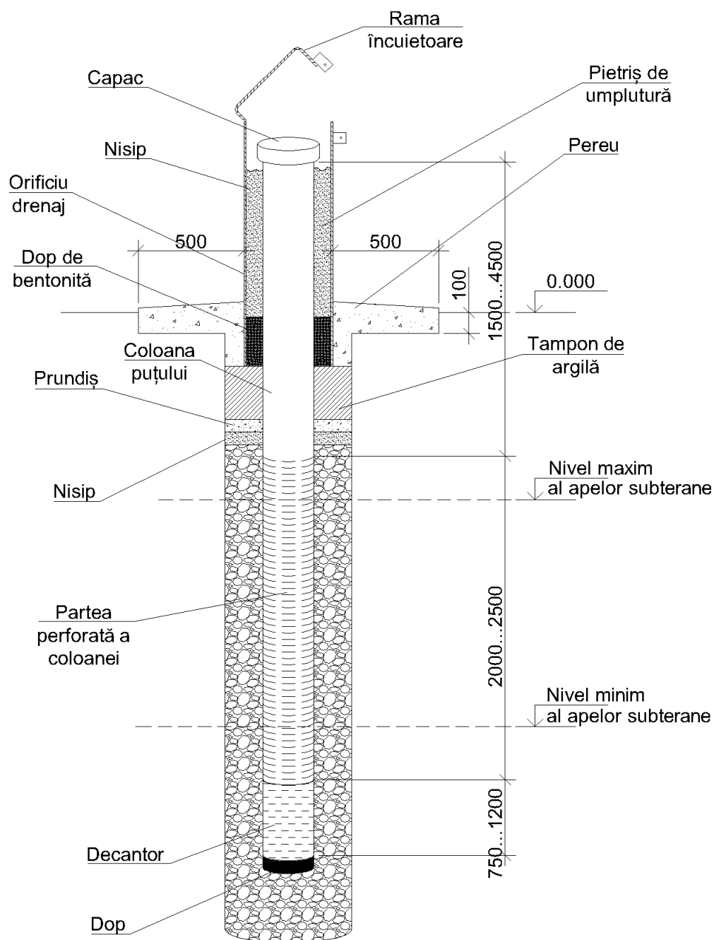
Figura 9 – Puț de control
