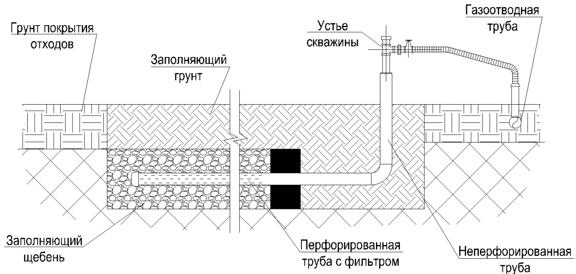
Рисунок 5 - Газосборный горизонтальный коллектор
