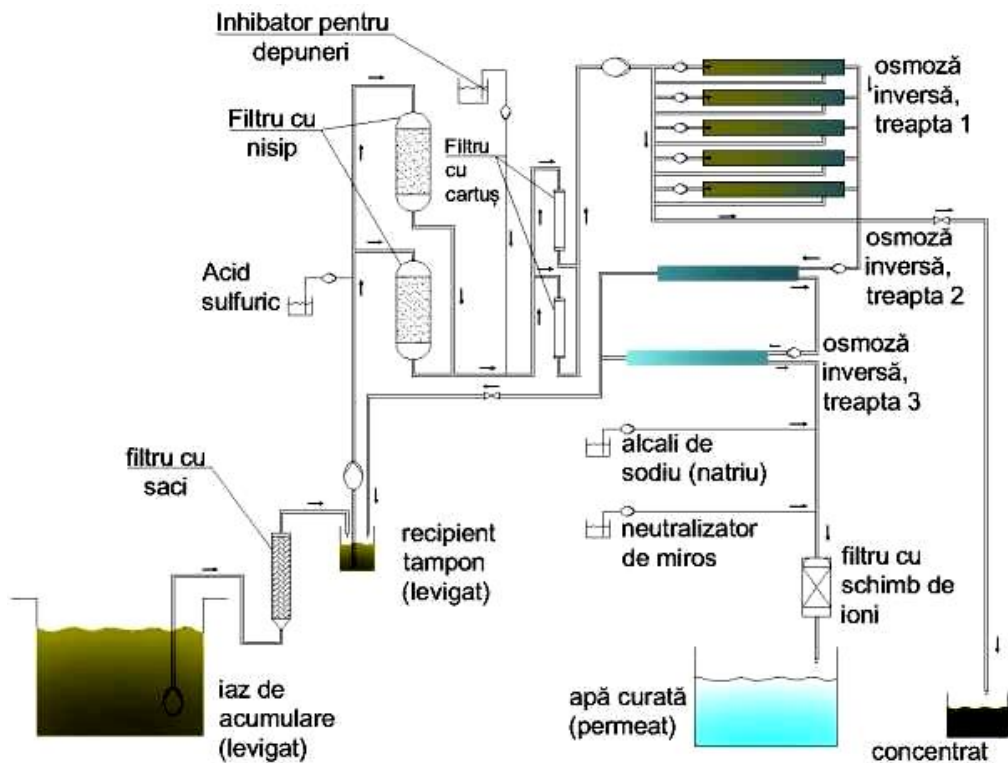
Figura 3 – Schema tehnologică a instalației de osmoză inversă pentru curățarea levigatului de la depozitul de deșeuri
