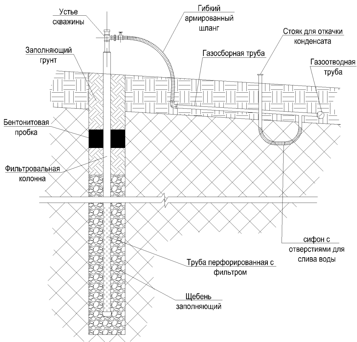
Рисунок 4 - Газосборная вертикальная скважина
