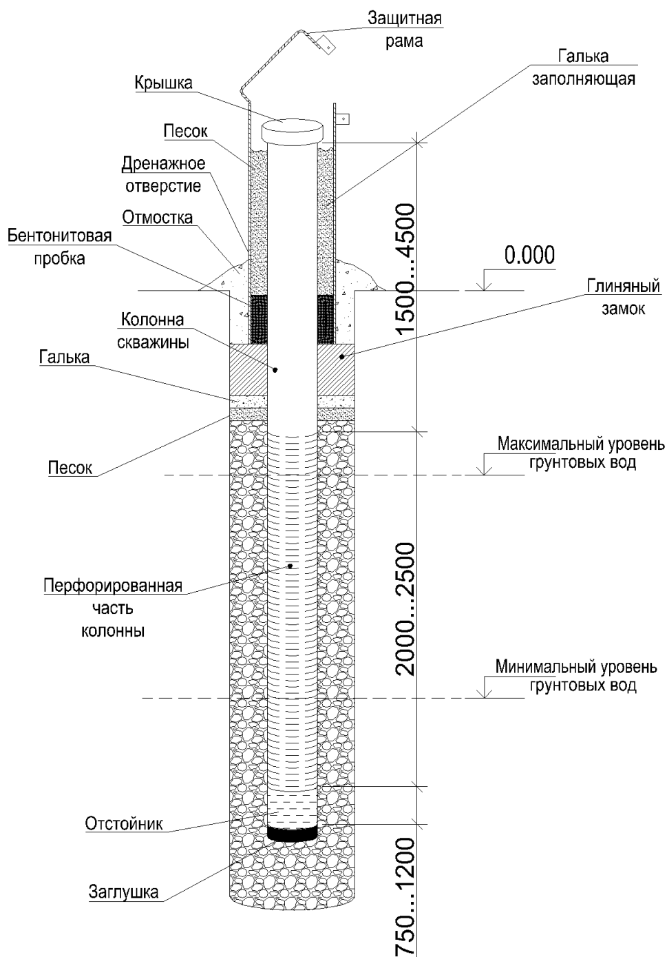
Рисунок 9 – Наблюдательная скважина
