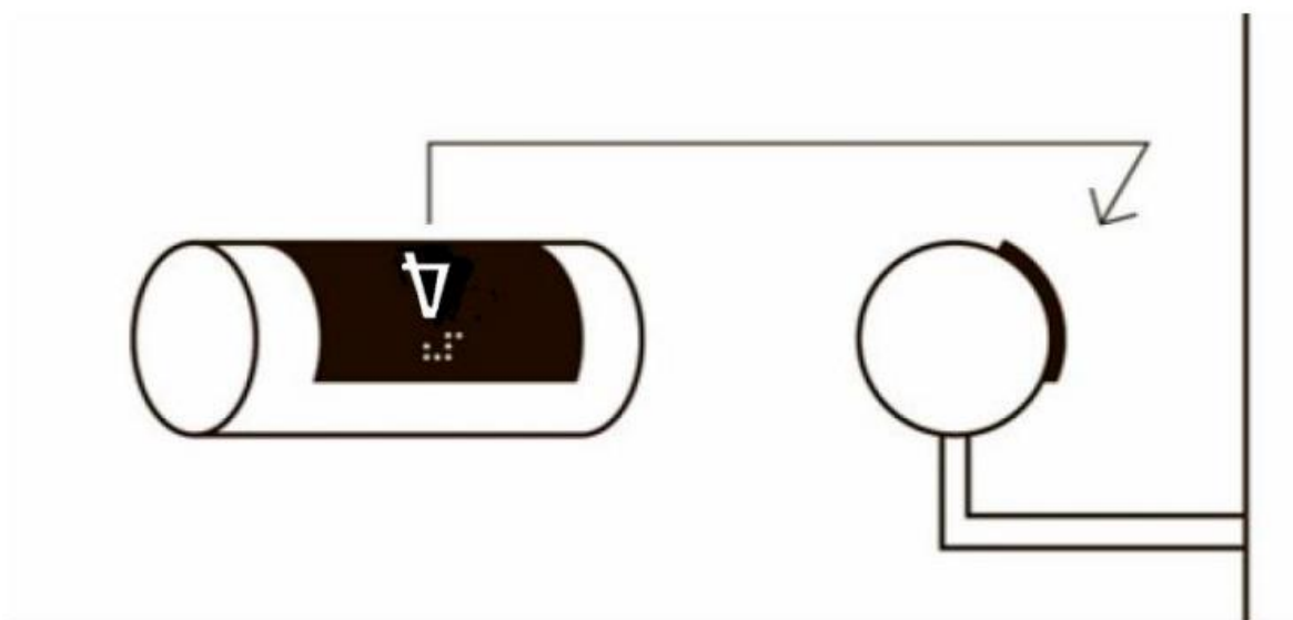
Figura 35 — amplasarea informației tactile pe mâinile curente (vedere a tăblii din partea peretelui)
