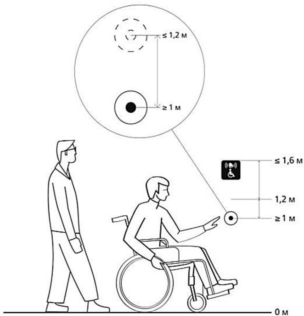
Figura 36 — Înălțimea de amplasare a butonului și tăbliei de informare
