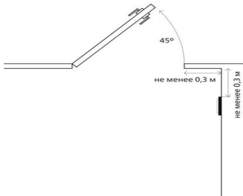
Рисунок 10 — Размещение информации при угловом расположении двери при затесненных условиях
