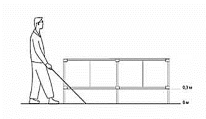
Figura C.3 — Îngrădiri cu înălțimea elementului de jos nu mai mare de 0.3 m
