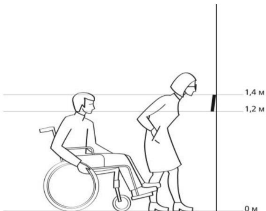
Рисунок 15 — Высота размещения информации для инвалида, использующего для передвижения кресло-коляску и углы обзора
