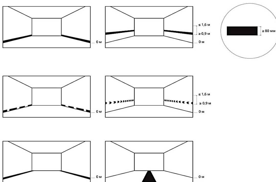
Figura 27 — Marcaj vizual de direcționare
