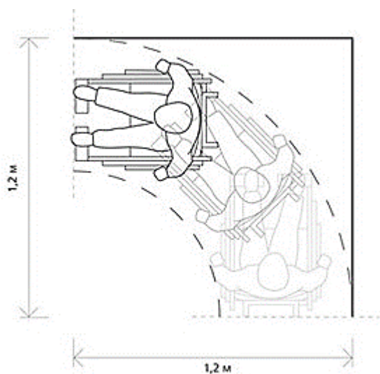
Figura B.2 — Spațiu pentru întoarcere la 90^\circ
