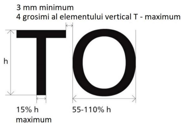
Figura 24 — Raportul dintre elementele semnelor fontului
