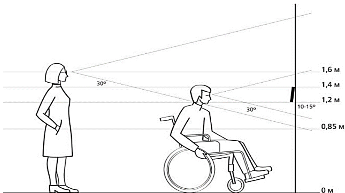
Figura 13 — Amplasarea informației pe plan vertical pentru persoana cu dizabilități care utilizează pentru deplasare scaun cu roțile
