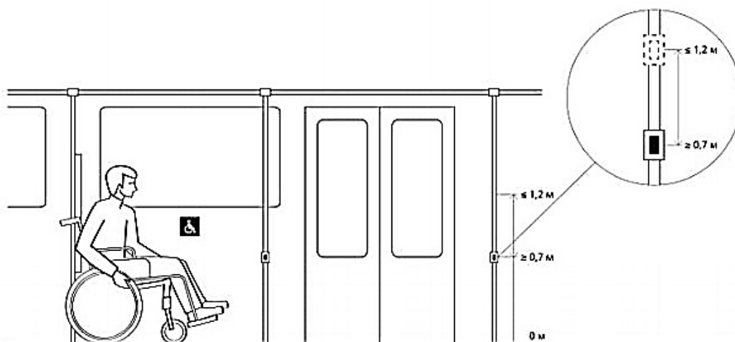
Figura 38 — Amplasarea butoanelor de apel al personalului pe mâinile curente a unităților de transport
