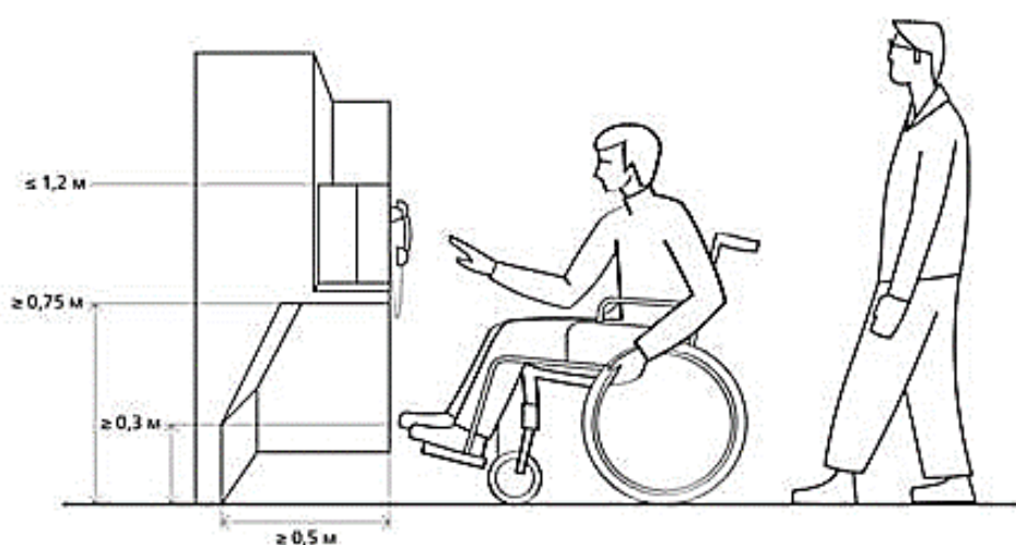
Figura B.5 — Adâncimea și înălțimea golului pentru picioare în cazul abordări frontale a utilajului
