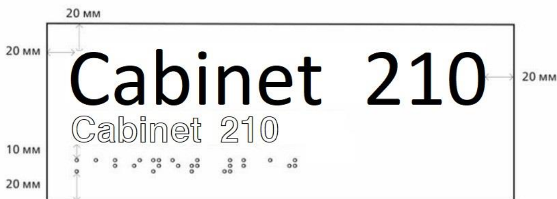
Figura 26 — Fundalul câmpului de lucru în raport cu granițele informației vizuale și tactile
