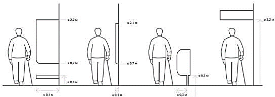
Рисунок С.2 — Выступы вдоль путей движения
