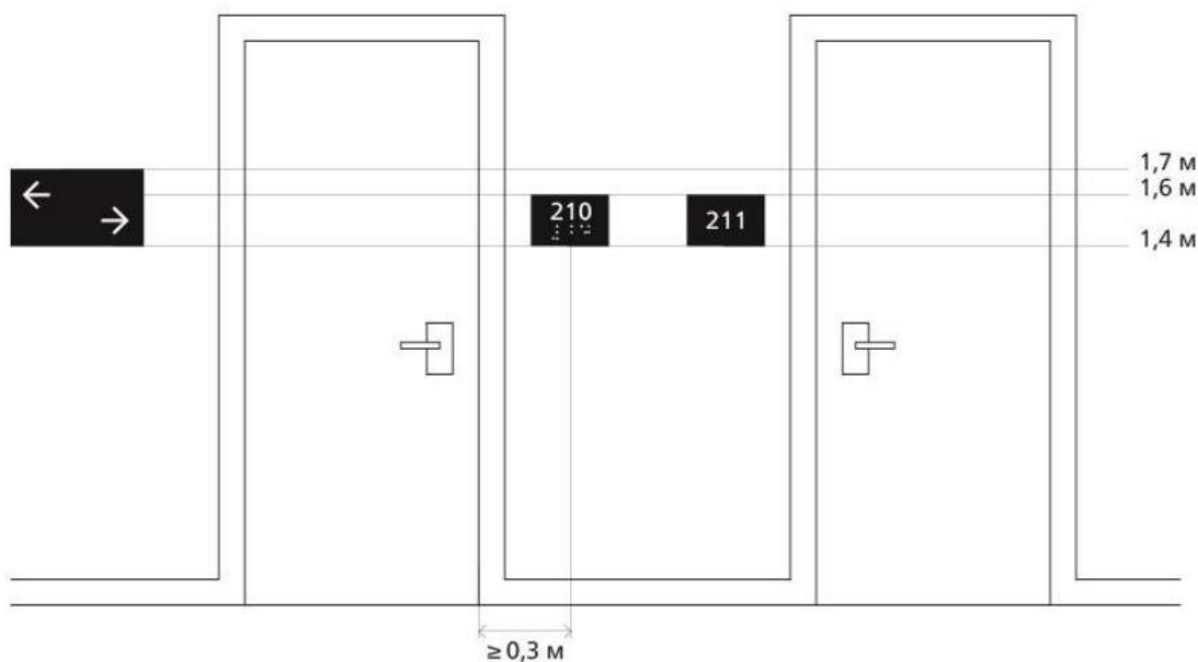
Рисунок 6 — Визуальная информация для идентификации помещений
