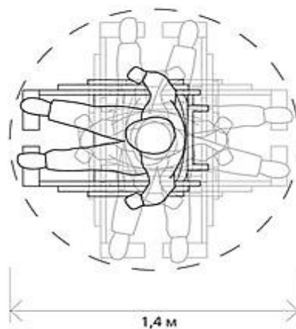
Figura B.3 — Spațiu pentru întoarcere în mod individual în orice direcție
