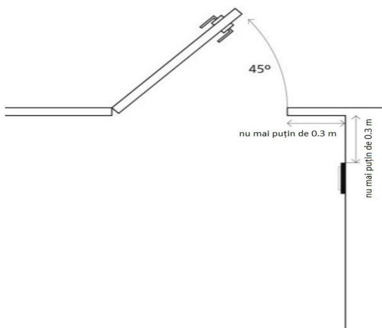
Figura 10 — Amplasarea informației în cazul amplasării în colț a ușii în condiții înghesuite
