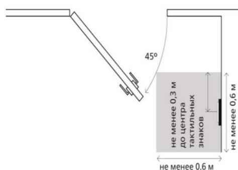
Рисунок 12 — Размещение информации при угловом расположении двери на расстоянии не менее 0.6 m от боковой стены
