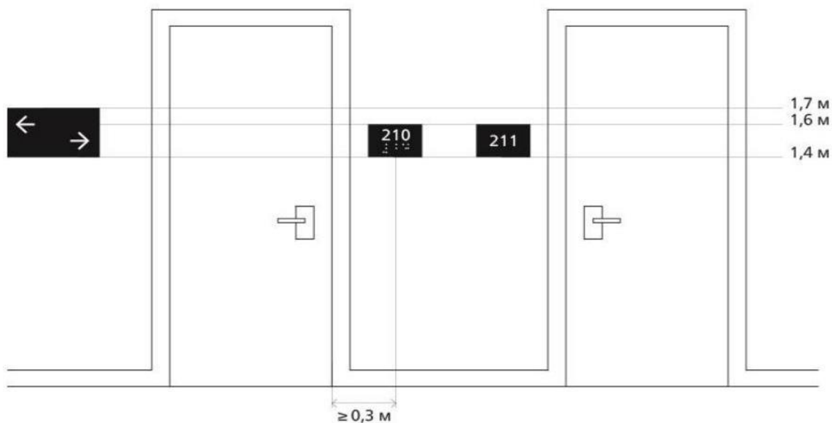
Figura 6 — Informația vizuală pentru identificarea încăperilor
