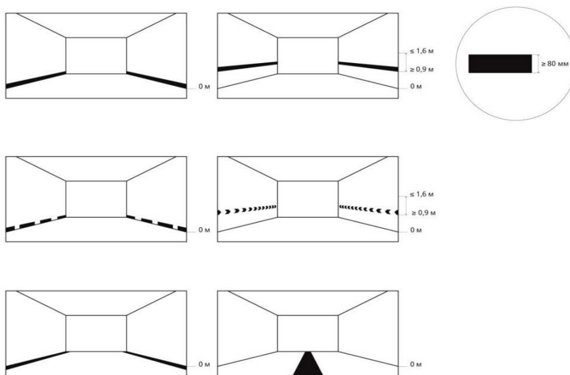
Рисунок 27 — Визуальная направляющая разметка
