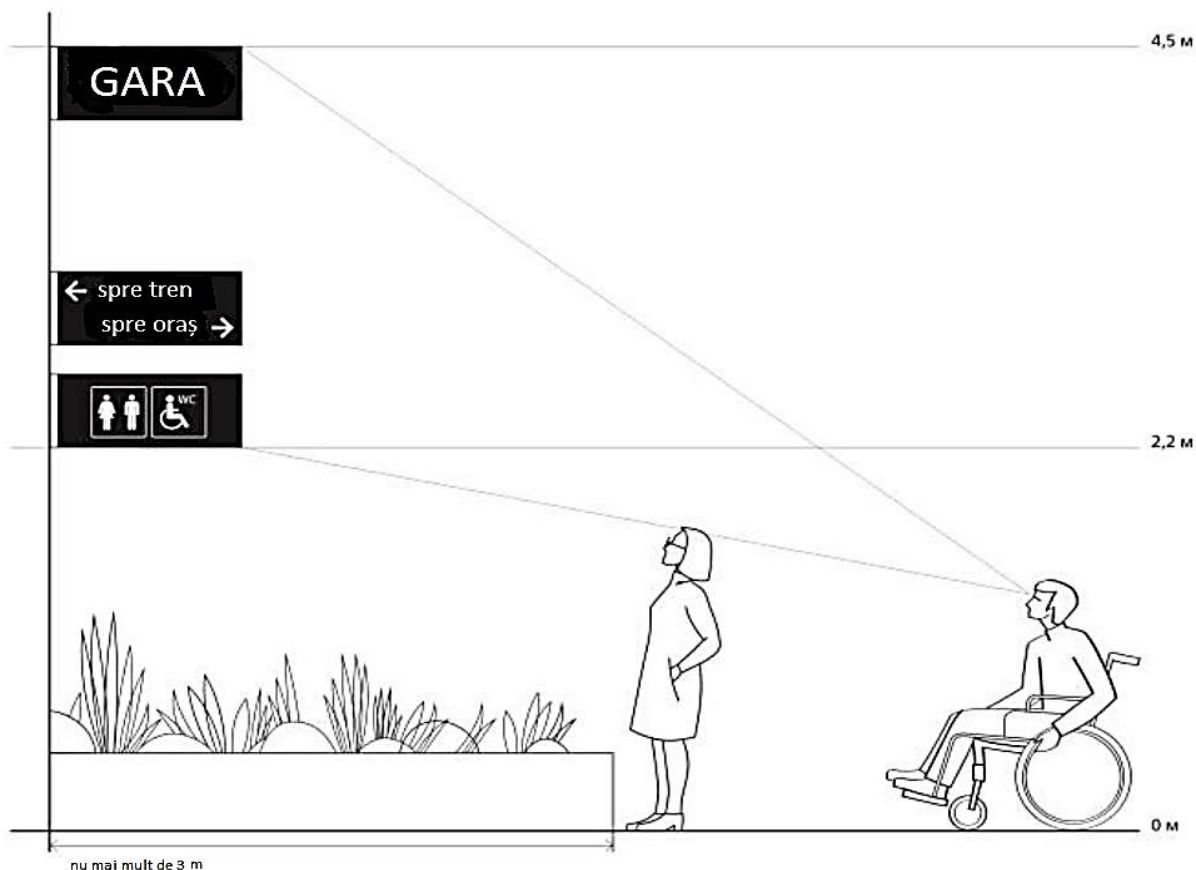
Figura 2 — Înălțimea amplasării mijloacelor de informare pentru orientare – a indicatorilor, amplasați pe console și pe console cu suspendare
