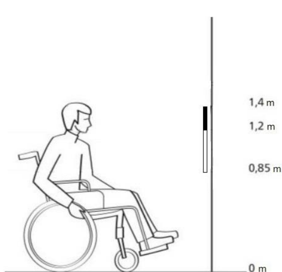
Figura 13 — Amplasarea informației pe plan vertical pentru persoana cu dizabilități care utilizează pentru deplasare scaun cu roțile
