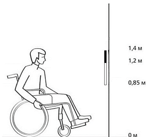
Рисунок 13 — Размещение информации на вертикальной плоскости для инвалида, использующего для передвижения кресло-коляску
