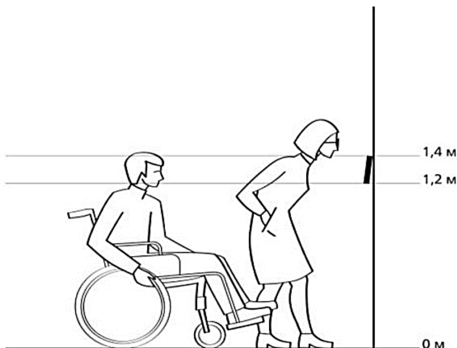
Figura 16 — Amplasarea informației sub unghi asigură vedere confortabilă pentru persoane cu dizabilități de toate categoriile
