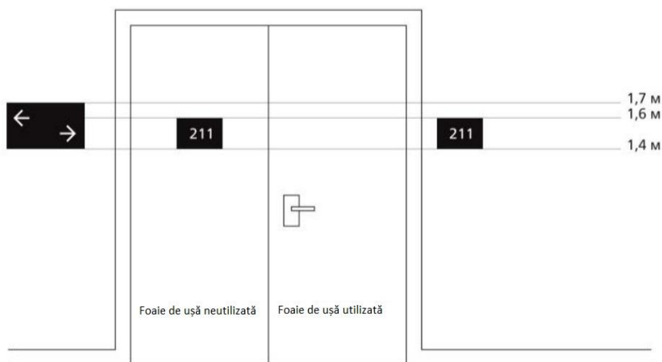
Figura 8 — Variantă de amplasare a informației pe tăbliile nefuncționale ale ușii cu două canape
