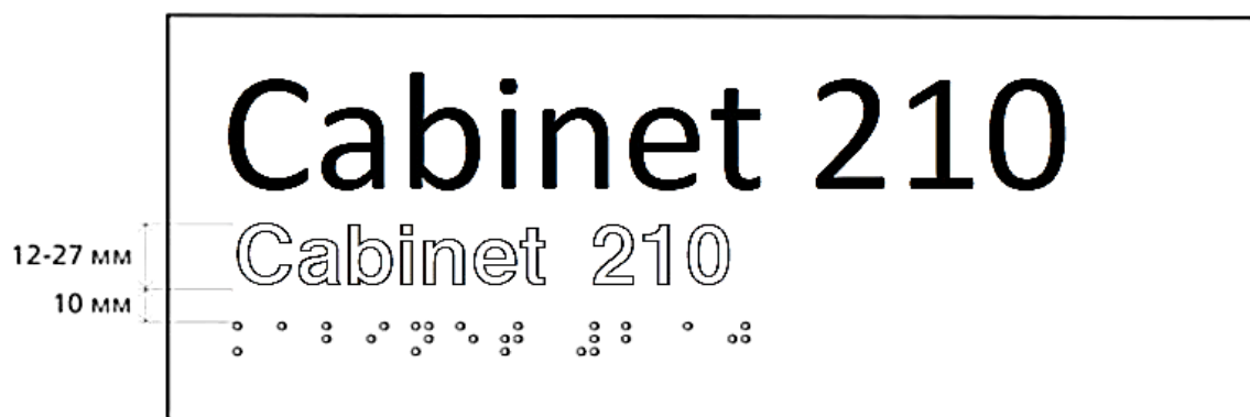
Figura 32 — Înălțimea FLR în combinație cu fontul tipărit plat (în acest caz semnele FLR și FPR se recomandă de executat transparente sau de culoarea fundalului)
