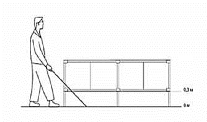
Рисунок С.3 — Ограждения с высотой нижнего элемента не выше 0.3 m
