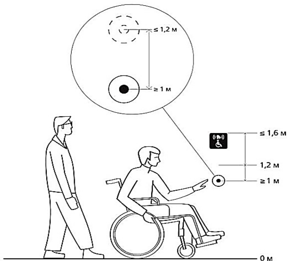
Рисунок 36 — Высота размещения кнопки и информирующей таблички
