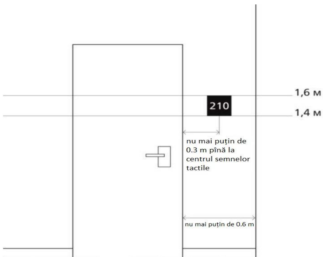
Figura 9 — Amplasarea informației relativ cu tăblia ușii
