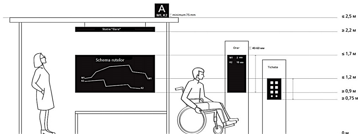
Figura 29 — Parametri de amplasare a mijloacelor de informare la stații
